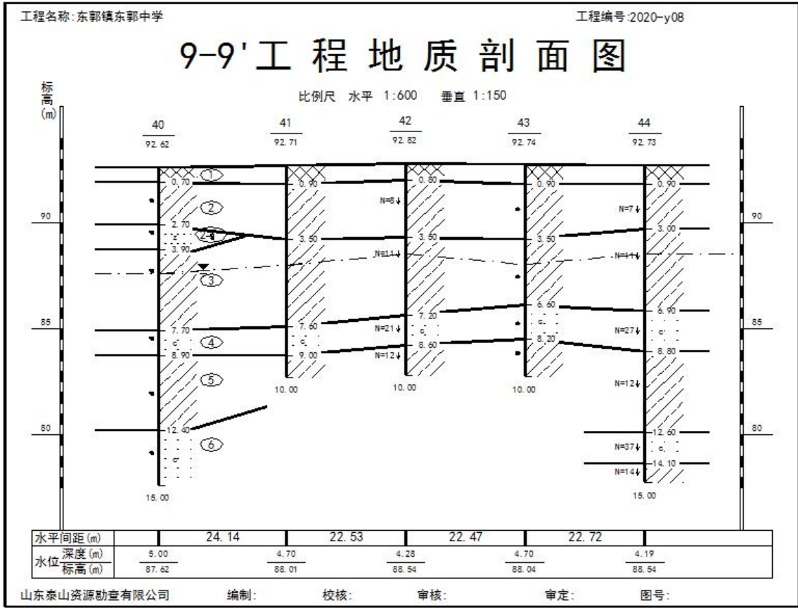
图 3-3 剖面图
