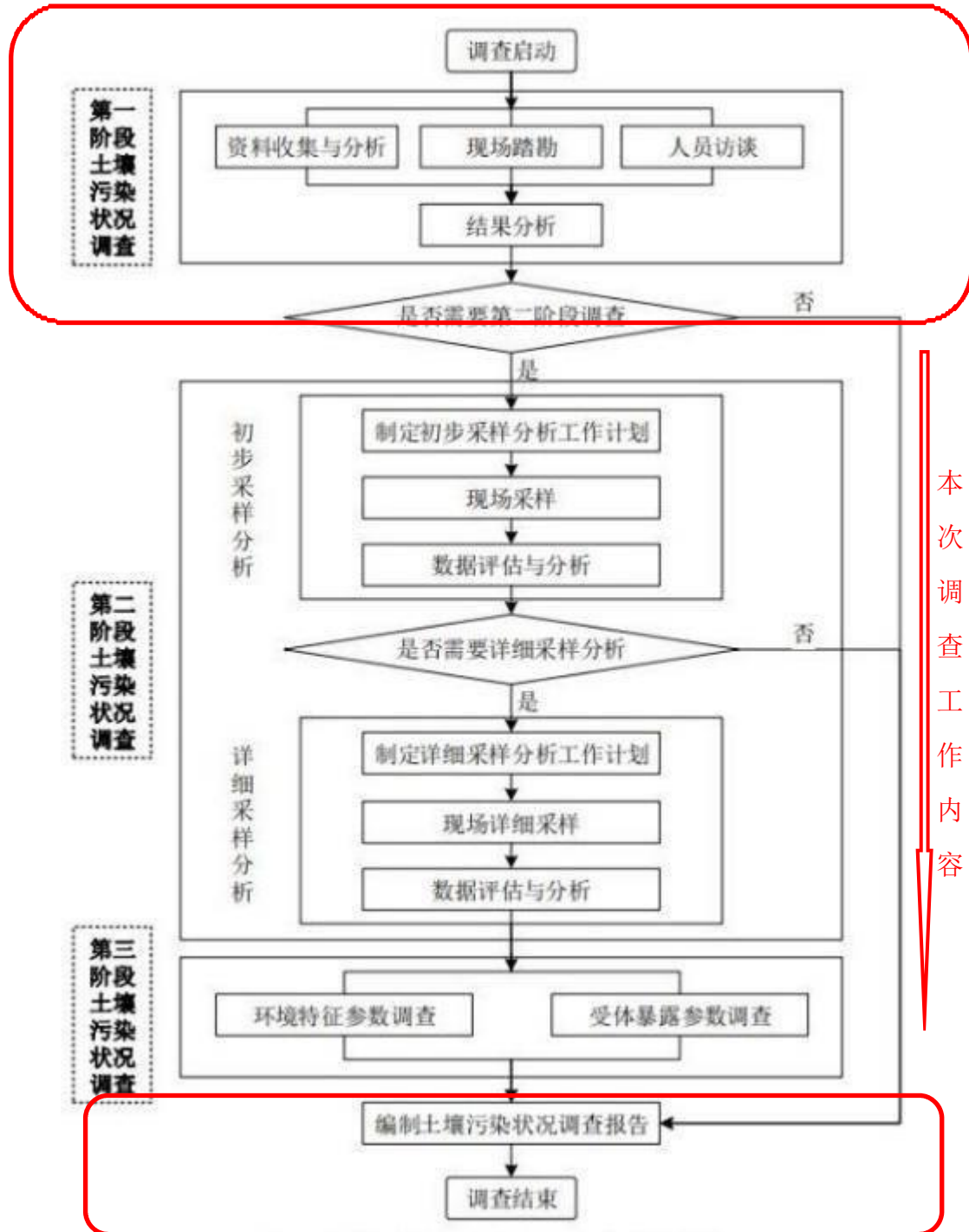
图 2-3 地块土壤污染状况调查的工作方法和程序
