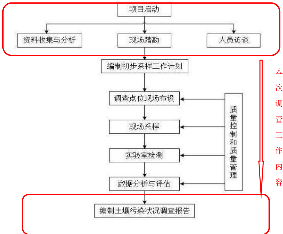
图2-4 地块土壤污染状况初步调查技术路线
