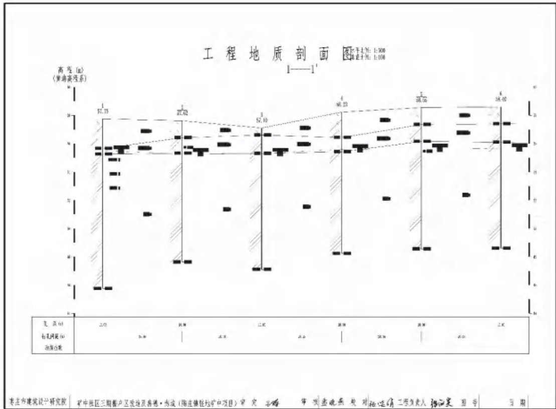
图 3.2-3 地质剖面图
